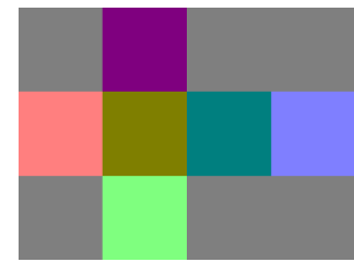
Würfel-Normalen
