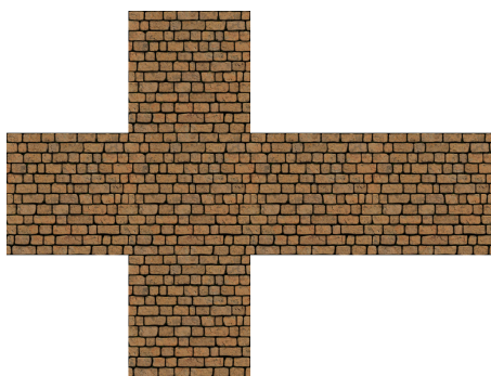
Würfel-Textur
